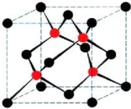
Diamante
