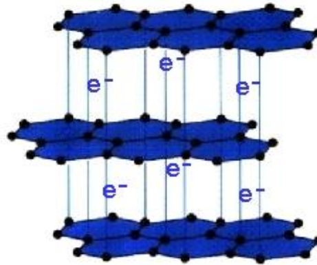
Grafito
